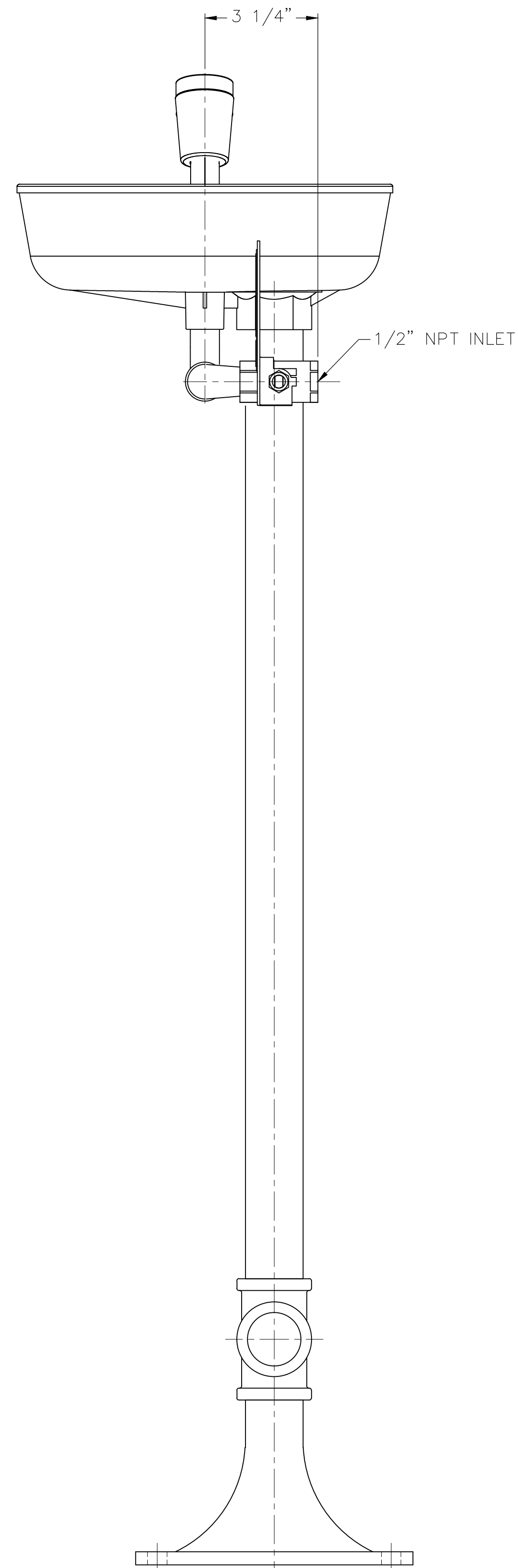
VIEW A-A
